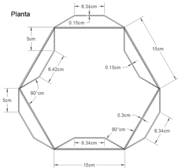
Junta para chaflán
